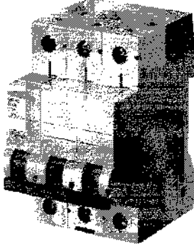
63 AMPER; 3 FAZLI; 70 mm; 6kA; C TİPİ; YAVAŞ KARAKTERLİ
